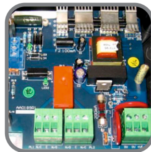
CIRCUIT IMPRIMÉ D'ALIMENTATION CC
