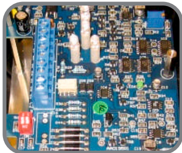
CIRCUIT IMPRIMÉ DE CONTRÔLE
